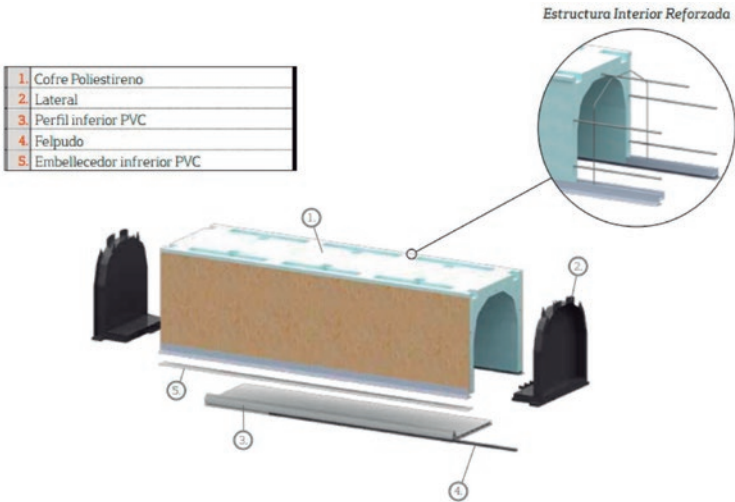
Figura 74. Partes del cajón túnel
