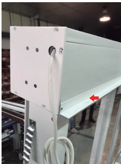
Figura 43. Tapajuntas en cajón
