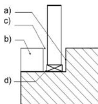
Figura 26. Definición de un galce de acristalamiento
